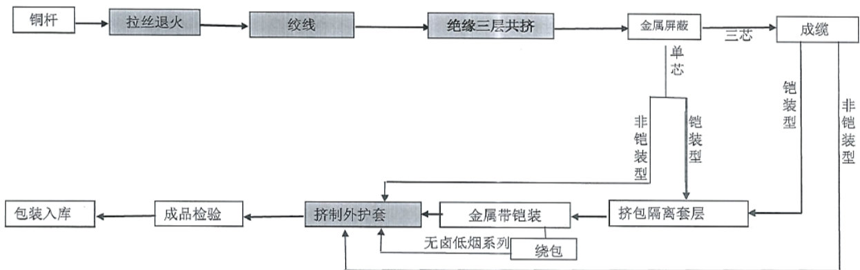
图3-1 生产工艺流程图
